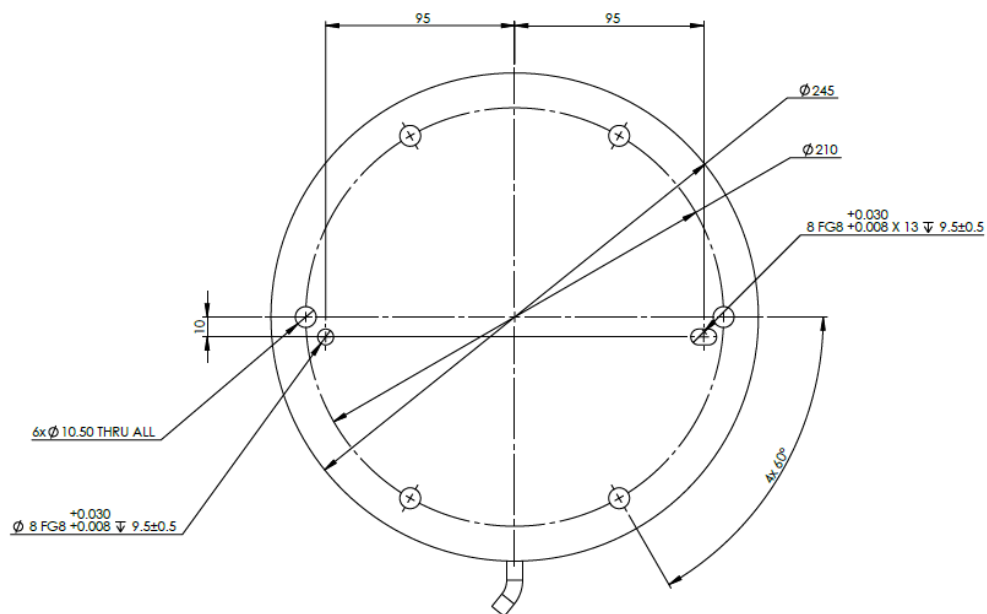
1.1: Vista dal basso della base del robot
